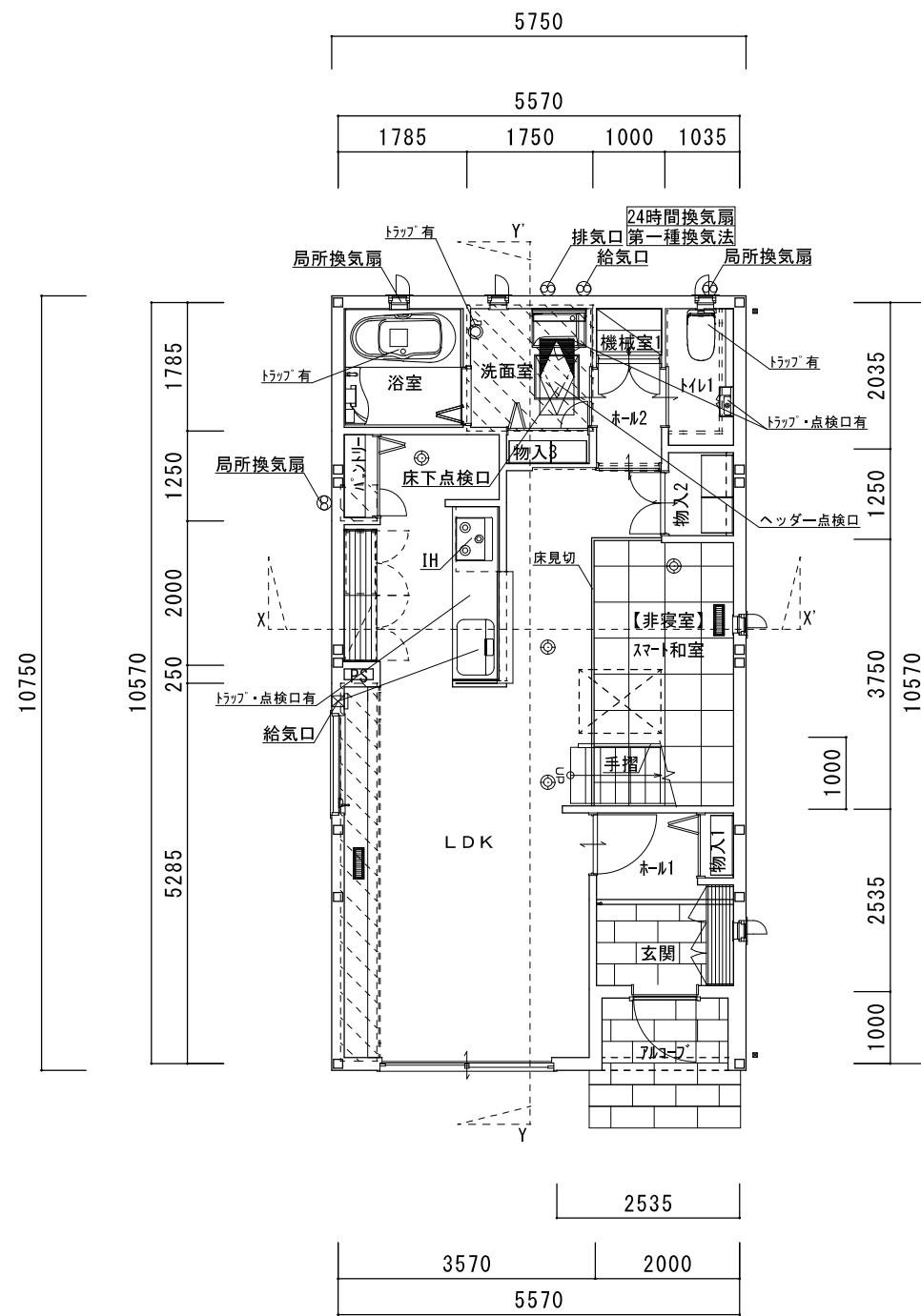
1階平面図
