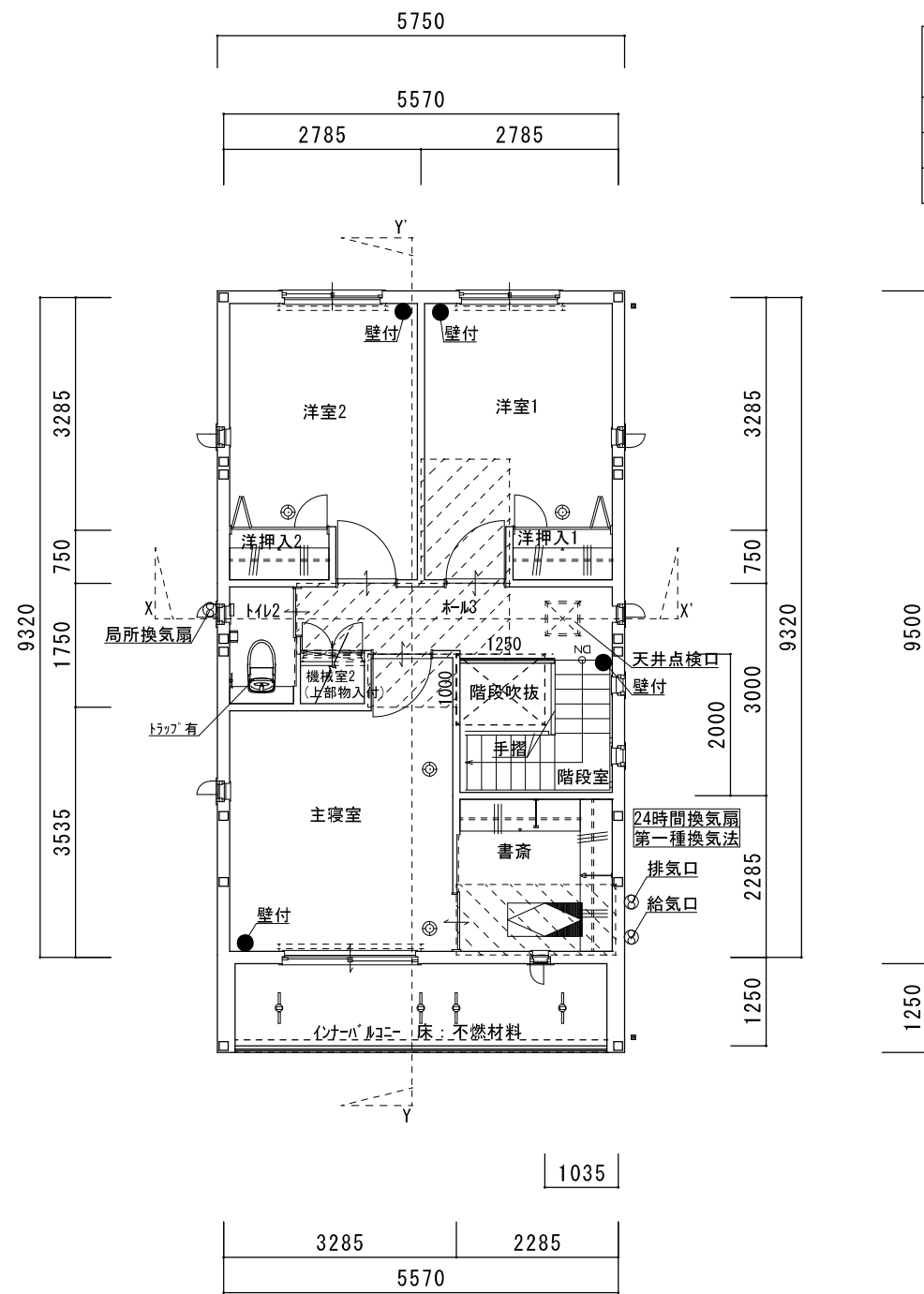
2階平面図
